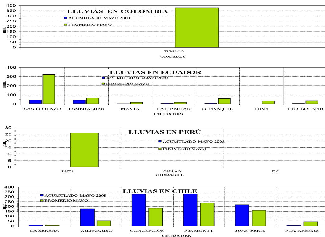
Figura 10.- Lluvia durante mayo en las estaciones costeras de Colombia, Ecuador, Perú y Chile. La ubicación de las estaciones se muestra en la Figura 1. (Fuentes: CCCP, INOCAR, DHN y DMCh).
