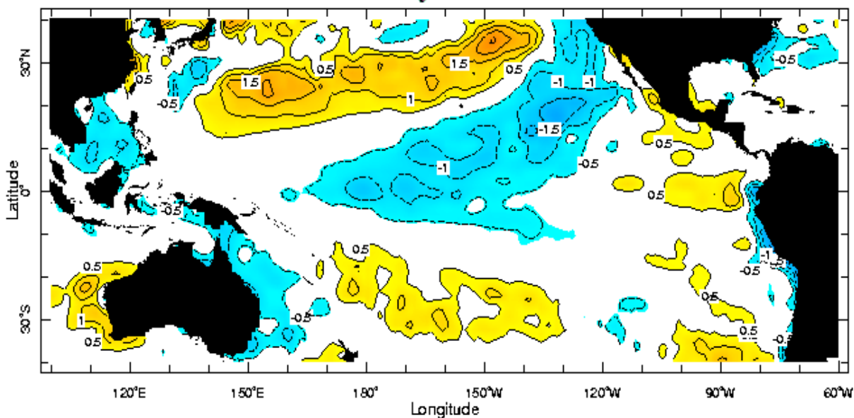
Figura 11.- Anomalia de la temperatura superficial del mar (°C) para mayo de 2008. (Fuente: International Research Institute for Climate and Society)
